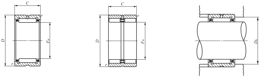
RNA49 TAF TR RNA69 ( F w ≤ 35) GTR
